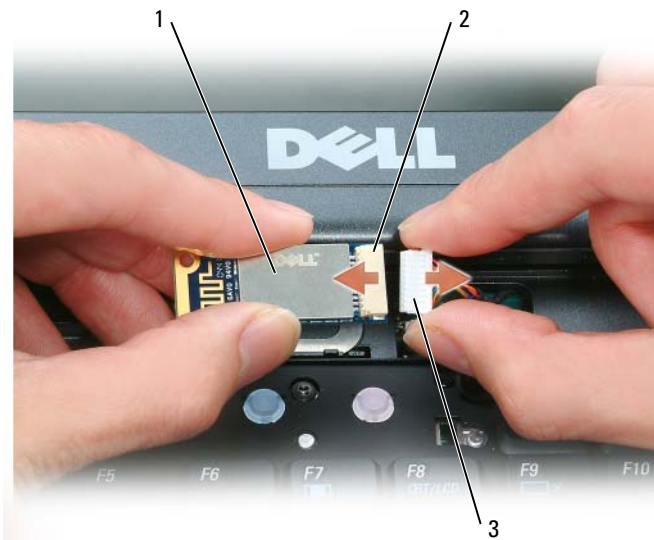
1 插卡 2 插卡連接器 3 纜線連接器
